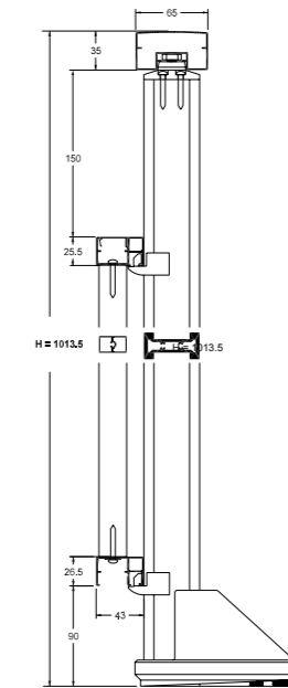
BARREAUDAGE DEVANT POTEAUX
