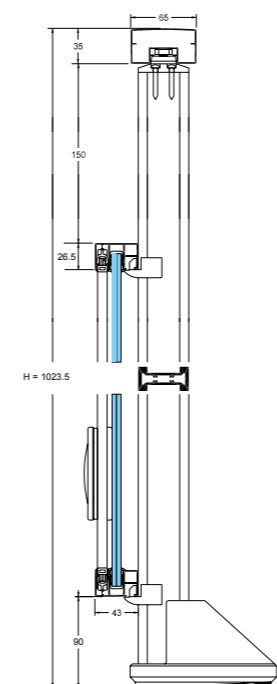
BANDE FILANTE CROIX DE SAINT-ANDRÉ
