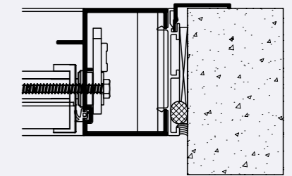
Coupe horizontale
