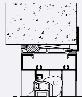
Coupe supérieure
