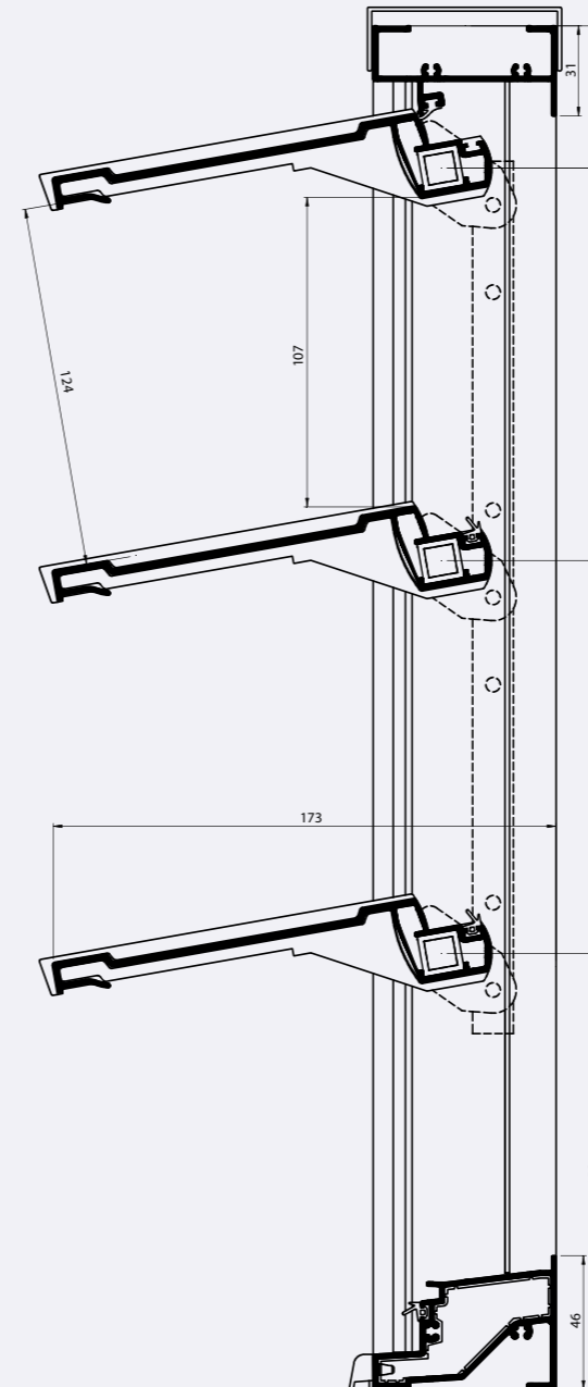
Coupes verticales
