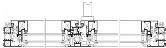
Coupe horizontale du système testé
