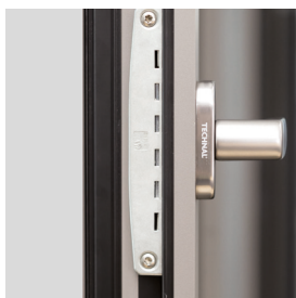
Manœuvre des fermetures par boîtier crémonne bidirectionnel
